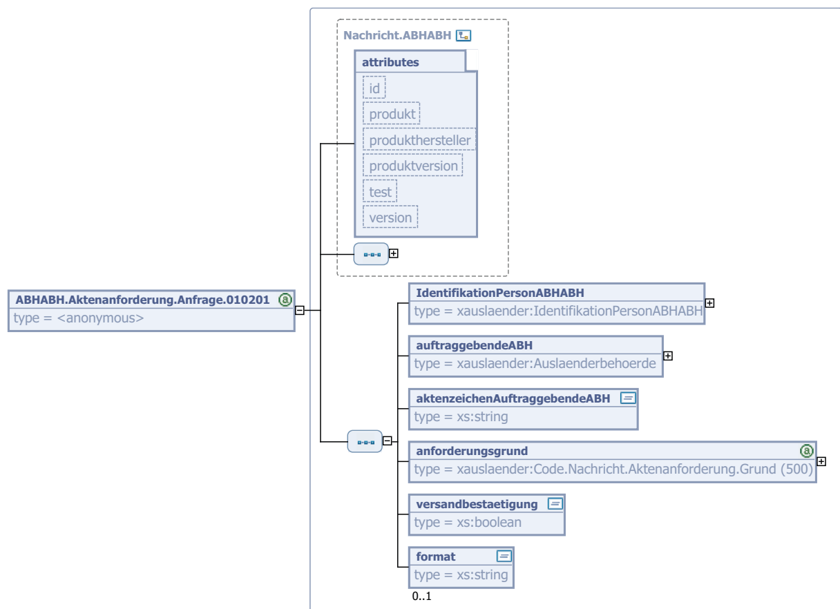
Bild 5-10 ABHABH.Aktenanforderung.Anfrage.010201
