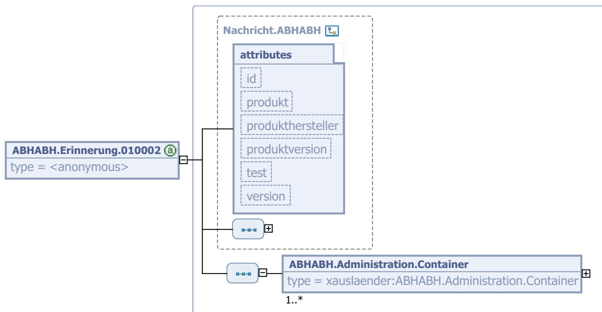
Bild 4-3 ABHABH.Erinnerung.010002
